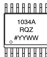
QSOP-16 CASE 492
