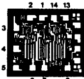
SCL4025B 51 x 44 mils
