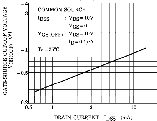
V_{GS}(\text{OFF}) - I_{DSS}
