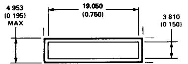
TOP B
