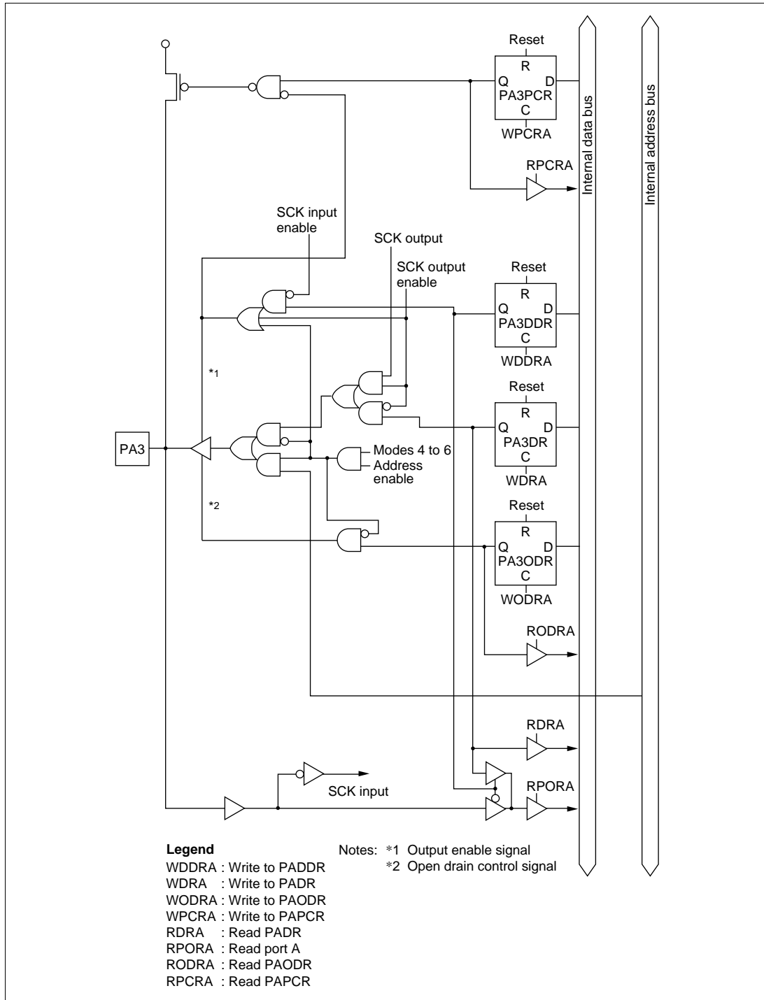
Figure C-6 (d) Port A Block Diagram (Pin PA3)
