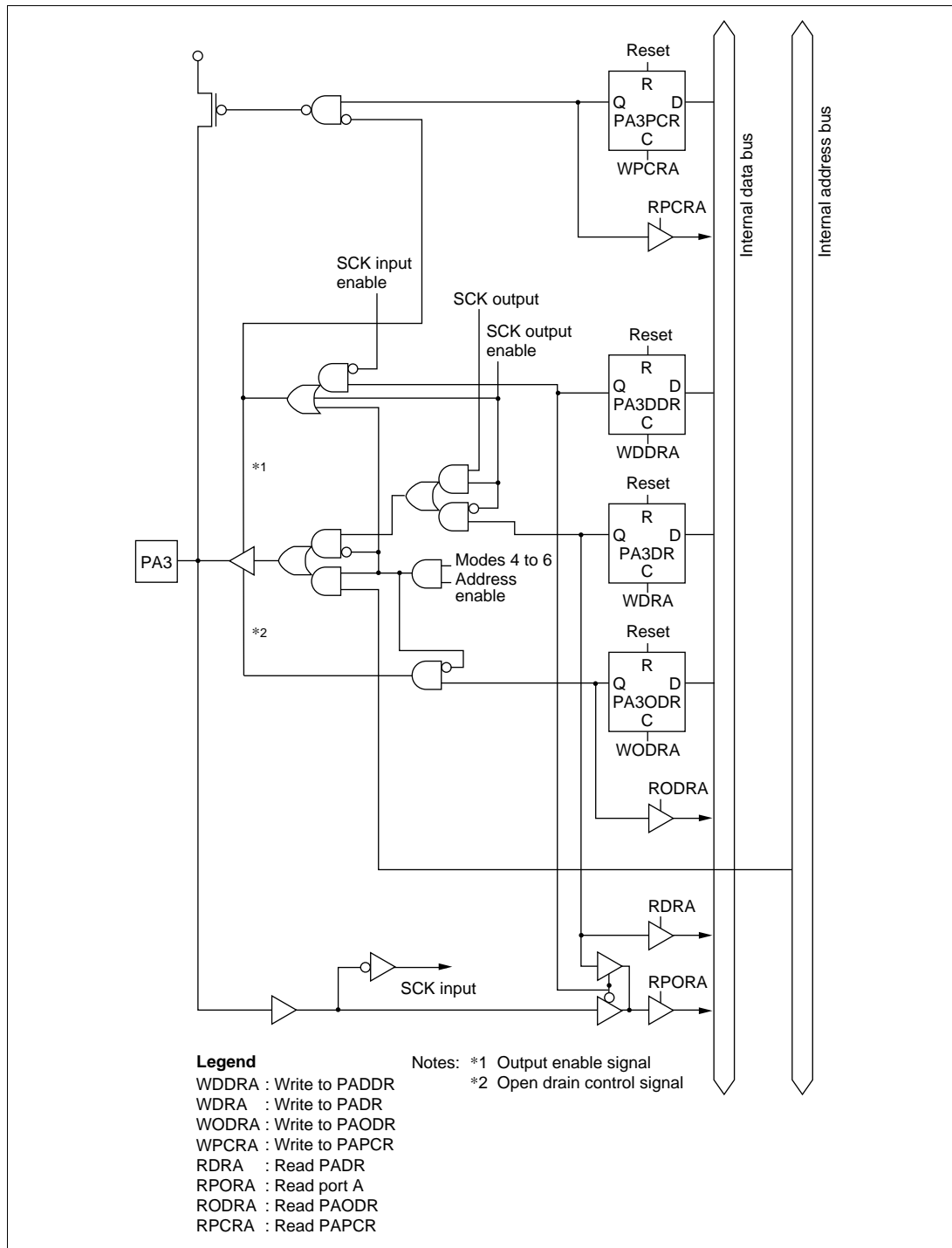
Figure C-18 (d) Port A Block Diagram (Pin PA3)
