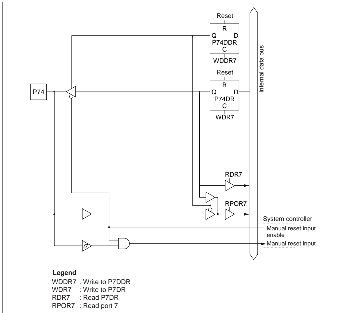
Figure C-16 (d) Port 7 Block Diagram (Pin P74)
