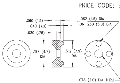
400-100
