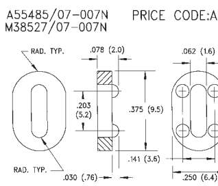
420-078
