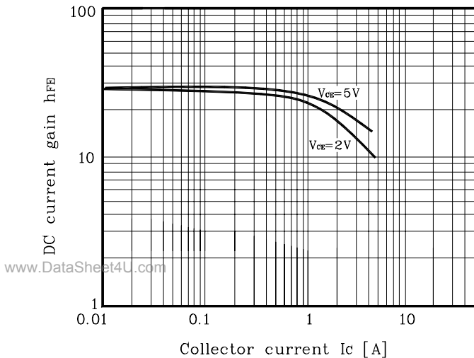
Fig. 3 h_{FE} - I_C
