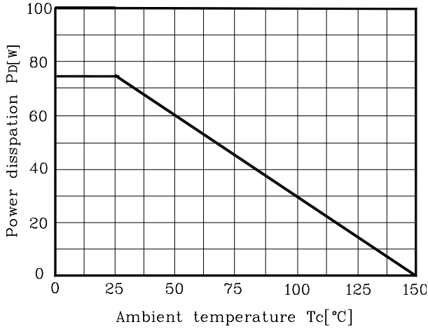
Fig. 1 P_D - T_C
