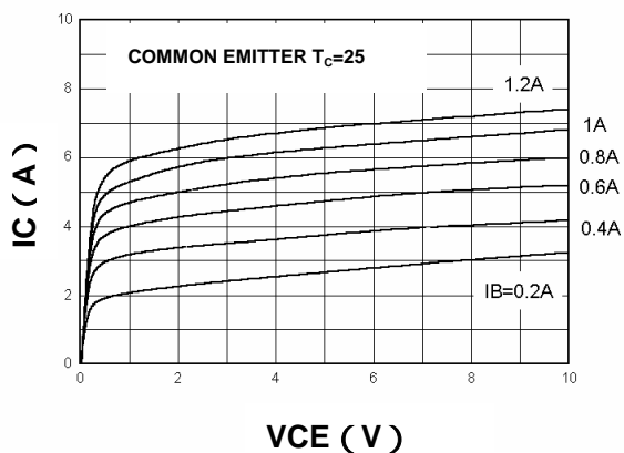
IC - VCE
