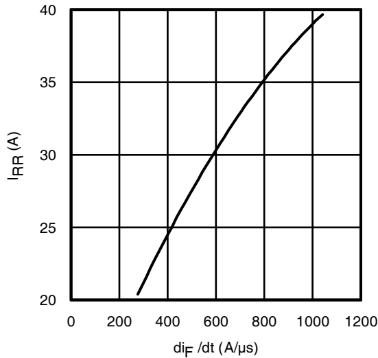
Fig. 19 - Typ. Diode I_{RR} vs. di/dt V_{CC} = 600\text{V} ; V_{GE} = 15\text{V} ; I_F = 30\text{A} ; T_J = 150^\circ\text{C}
