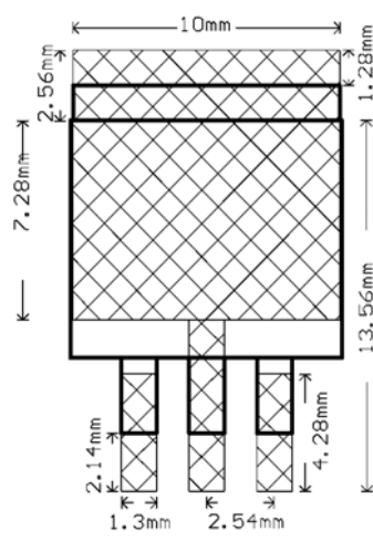
TO-263T
