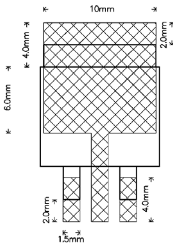
TO-263
