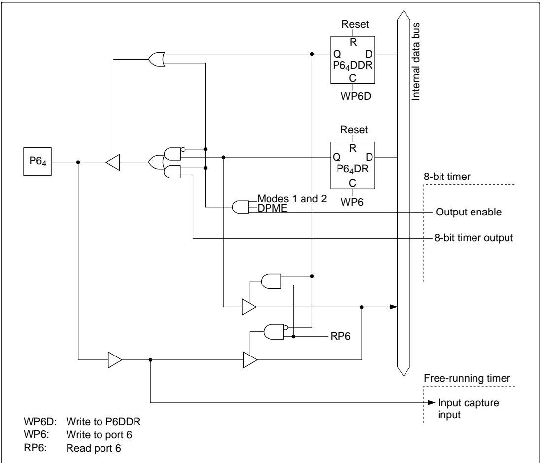
Figure C.6 (d) Port 6 Block Diagram (Pin P6 4 )
