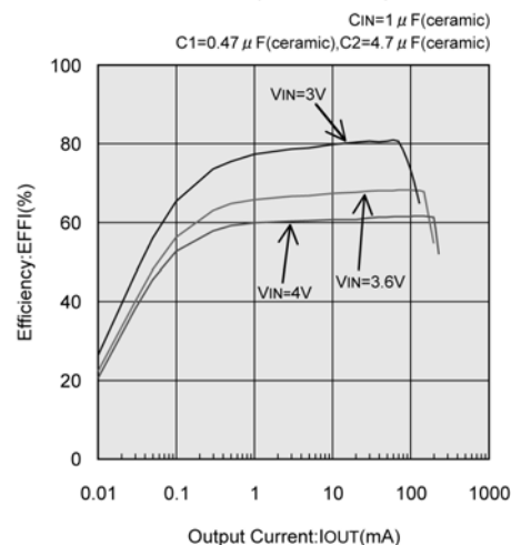
XC9802B503KR(300kHz,5.0V)
