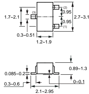
SC-59/SOT-346
