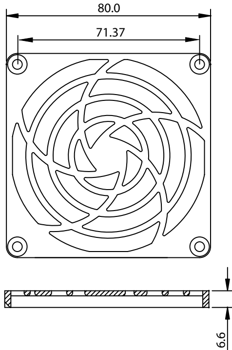
FAN GUARD
