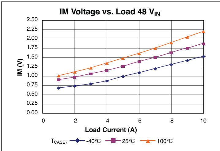
Figure 7 – IM voltage vs. load; 48 V_{IN}
