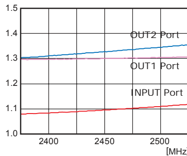
VSWR
