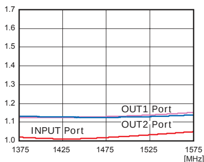
VSWR
