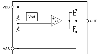
CMOS Output
