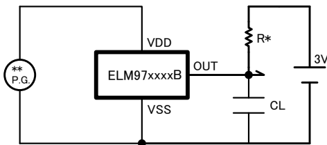
4) Delay time
