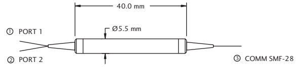
P2: 900µm loose tube
