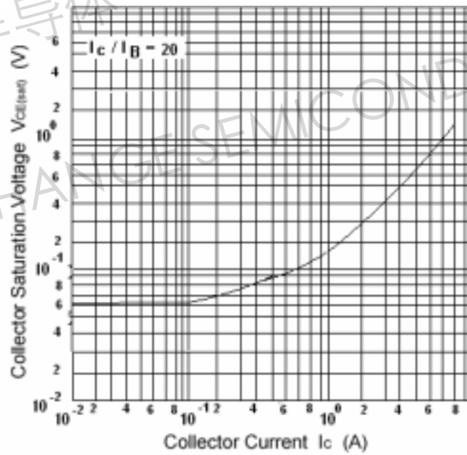
Fig.4 V_{CE(sat)} - I_C
