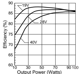
MFLHP2815S & MFLHP2815D Efficiency
