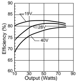
MFLHP2805S & MFLHP2805D Efficiency
