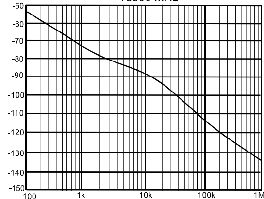
Phase Noise (dBc/Hz) 18500 MHz
