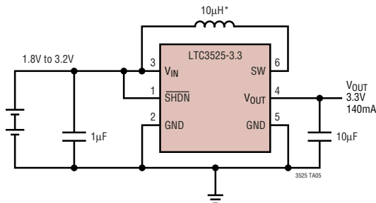
2-Alkaline or NiMH to 3.3V
