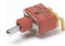
E101MD1ABE Horizontal Actuation SPDT
