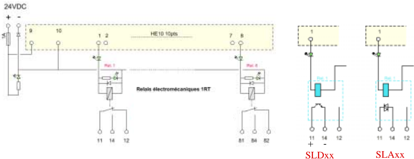
Schéma de principe / wiring diagram
