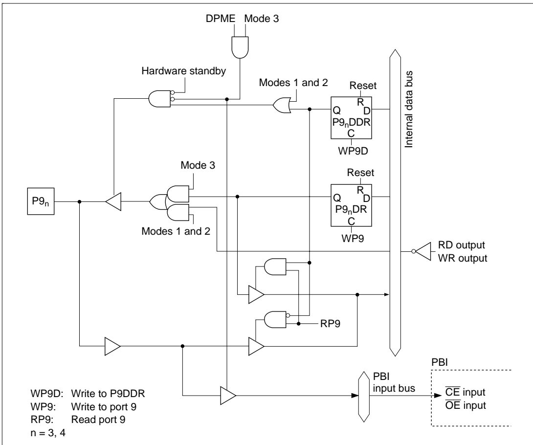
Figure C.9 (d) Port 9 Block Diagram (Pins P9 3 , P9 4 )
