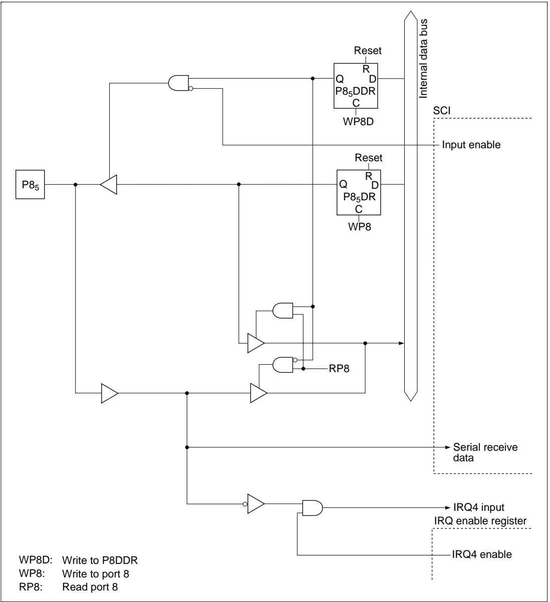
Figure C.8 (d) Port 8 Block Diagram (Pin P8 5 )
