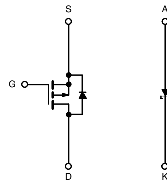
P-Channel MOSFET
