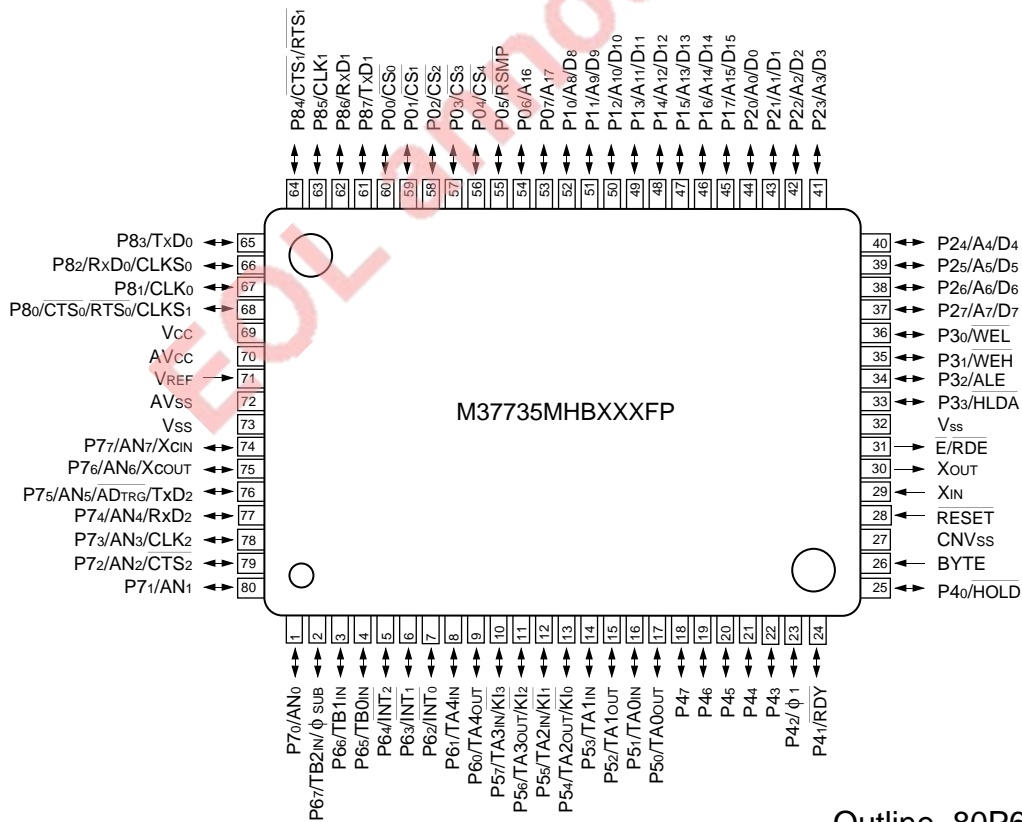
Outline 80P6N-A
