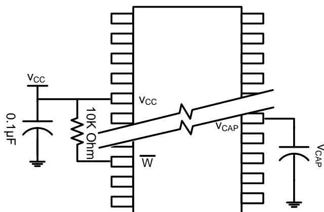
Figure 3: AutoStore Mode
