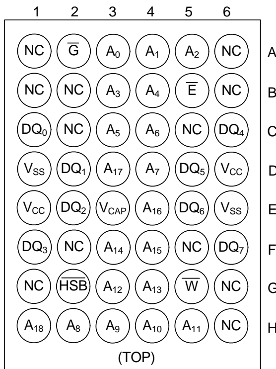
48-Ball FBGA
