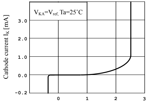
Fig.5 I_K vs V_{KA} (2)
