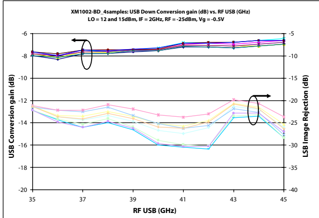
IF=2 GHz
