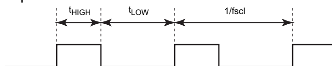
SCL output
