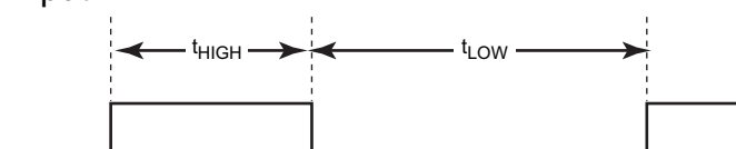
SCL input
