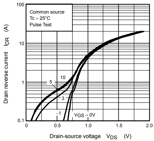
I_{DR} - V_{DS}
