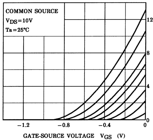
I_D - V_{GS}
