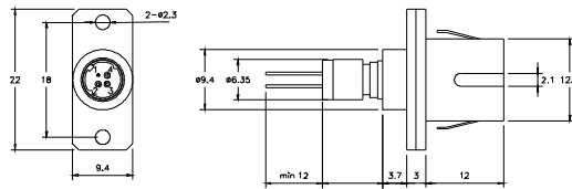
SC Receptacle
