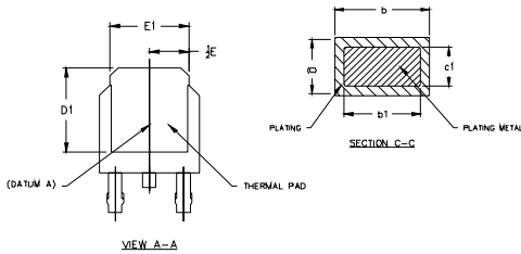
VIEW A-A
