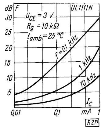
Współczynnik szumów w funkcji prądu kolektora ( R_g = 10 \text{ k}\Omega )
