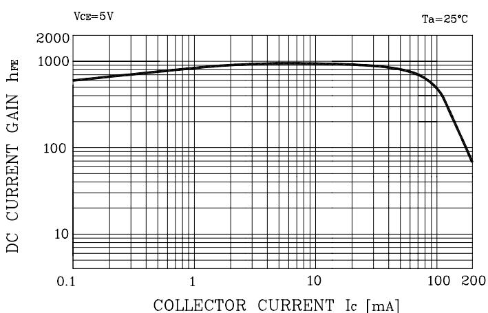
Fig. 1 h_{FE} - I_C
