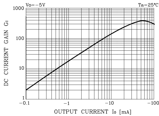
Fig. 3 G_I - I_O
