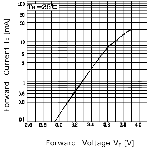
Fig. 1 I_F - V_F
