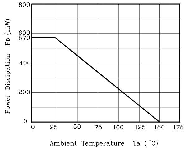
Fig. 4 P_D-T_a
