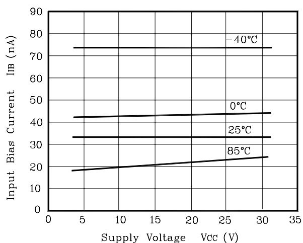
Fig. 2 V_{CC} - I_{IB}
