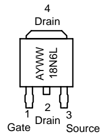
DPAK CASE 369C STYLE 2
