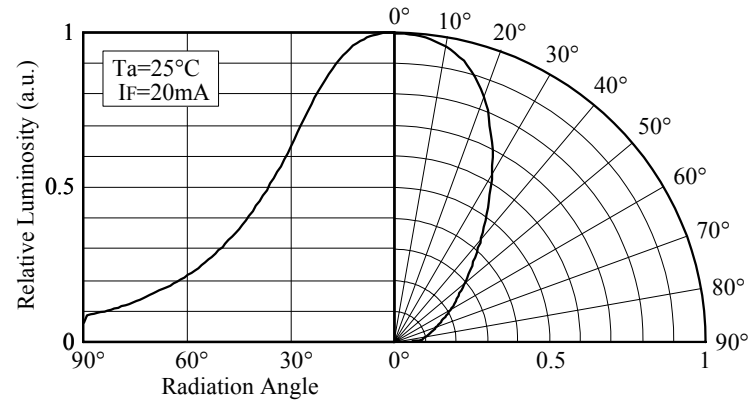
■ Directivity (NSPW515B(S))
