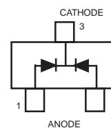
CASE 419-04, STYLE 5 SOT-323/SC-70
