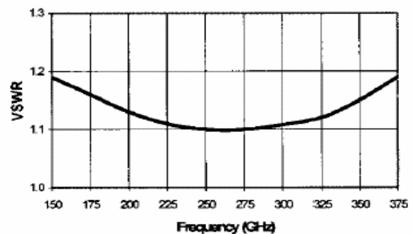
VSWR
