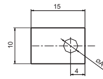
Style 077: A=Ø4.2 Style 077-1: A=Ø5.2 Style 077-2: A=Ø6.2
