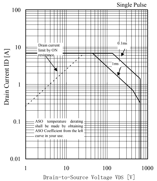
IRIS-G6651 MOSFET A.S.O. Curve T_a=25^\circ
