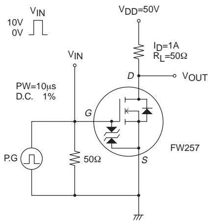
スイッチングタイム測定回路図
