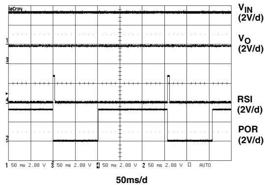
FIGURE 11. POR FUNCTION
