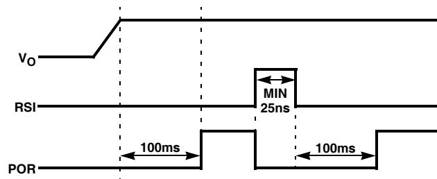
FIGURE 13. RSI & POR TIMING DIAGRAM
